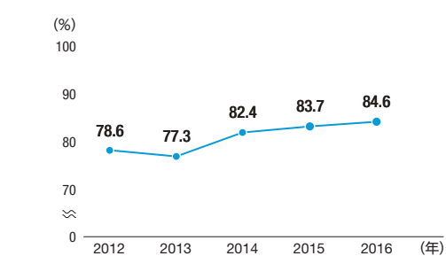
廃棄物リサイクル率(SUMCOグループ(国内))
