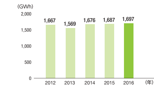
電力使用量(SUMCOグループ)
