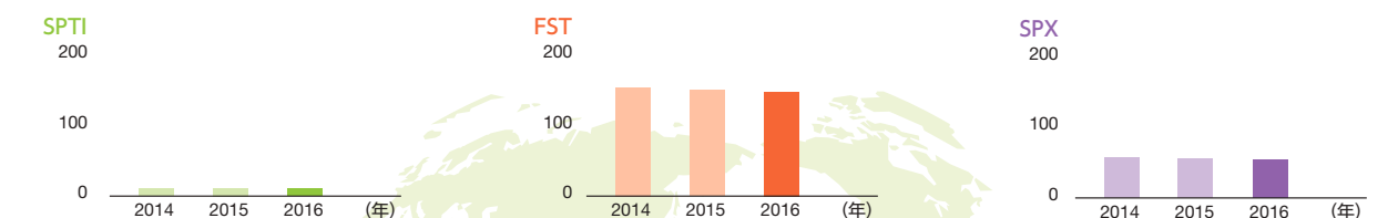
CO 2 排出量 推移 (海外) (千t-CO 2 /年)
