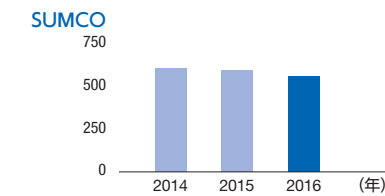
CO 2 排出量 推移 (国内) (千t-CO 2 /年)
