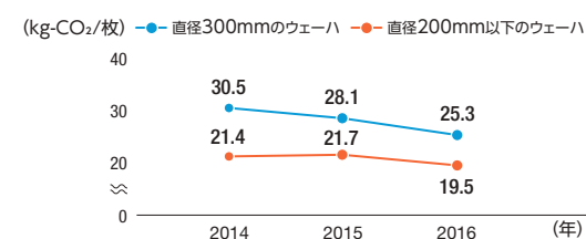
国内製品1枚あたりCO 2 排出量
