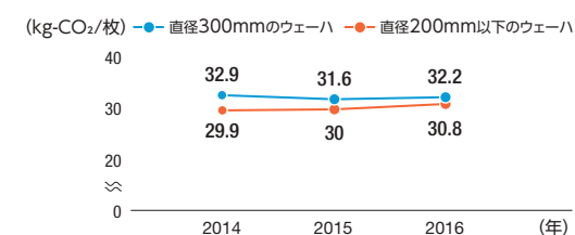
海外製品1枚あたりCO 2 排出量
