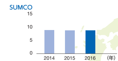
水使用量 推移 (国内) (Mm³/年)
